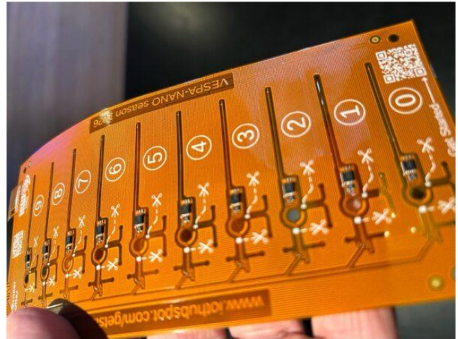
Figuur 2: blad met 10 vespa nano zenders, die bij gebruik worden lostgemaakt uit het blad
